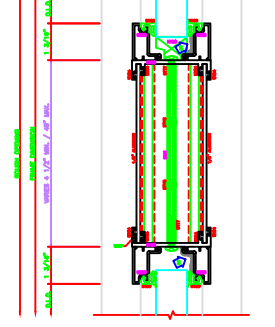
510 SIDE LITE HORIZ. 25/25/25/25
